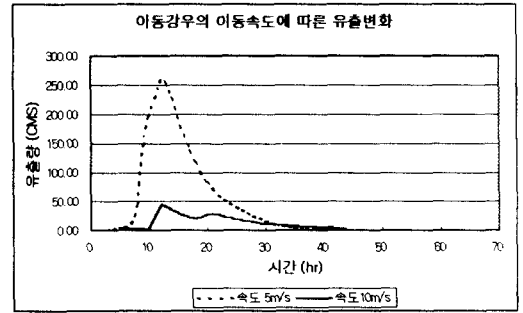
그림 10. 7번방향에서 이동속도에 따른 유출변화
