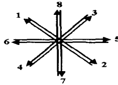
그림 4. 강우의 이동방향
