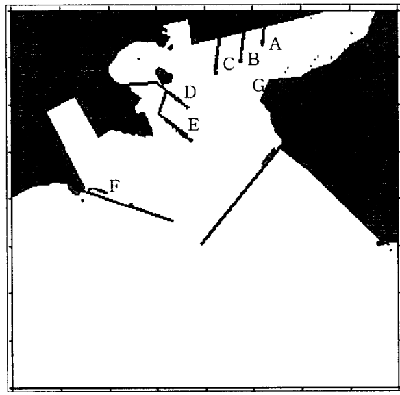
그림 2 항내 파고산정 구역도
