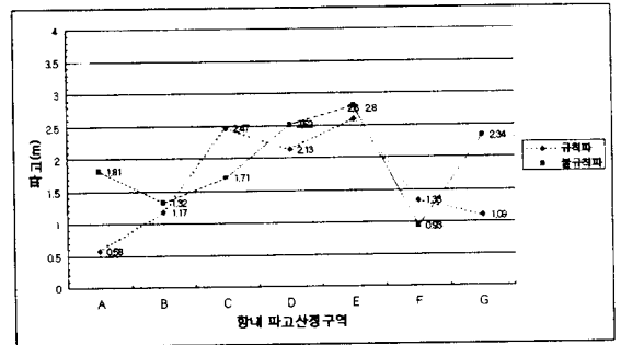
그림 8 CASE 2의 구역별 파고분포
