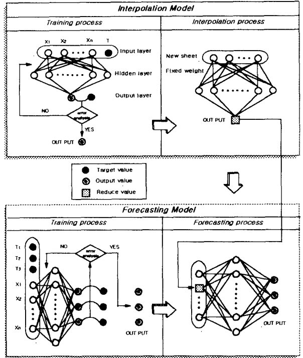
그림 2. 신경망모형의 연계모식도
