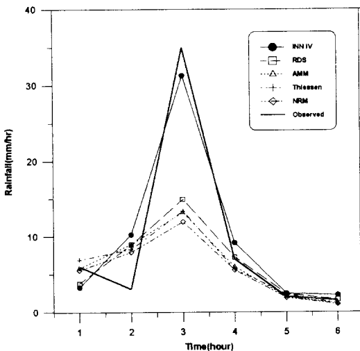
그림 4. 강우 결측보완 결과(1995.07.11)
