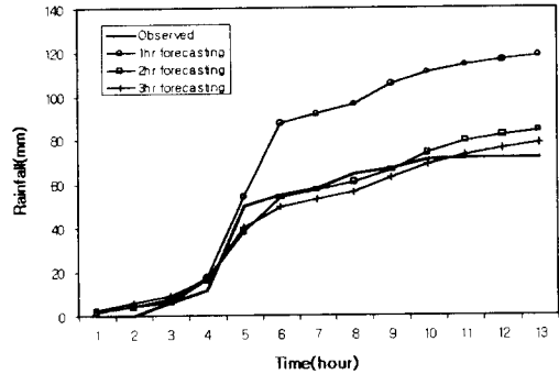
그림 7. 강우예측 누가우량 곡선(1997.07.01)
