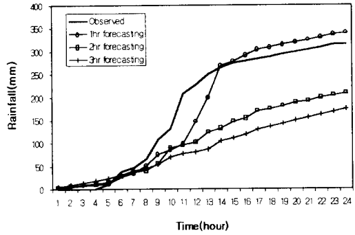
그림 9. 강우예측 누가우량 곡선(1998.08.11)
