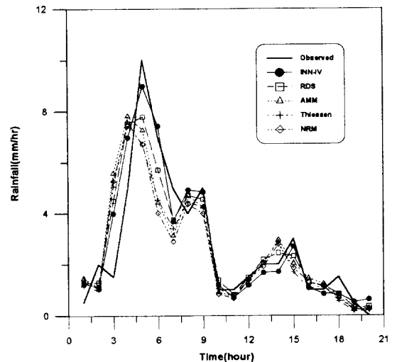
그림 5. 강우 결측보완 결과(1996.07.04)
