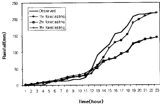
그림 8. 강우예측 누가우량 곡선(1997.08.03)
