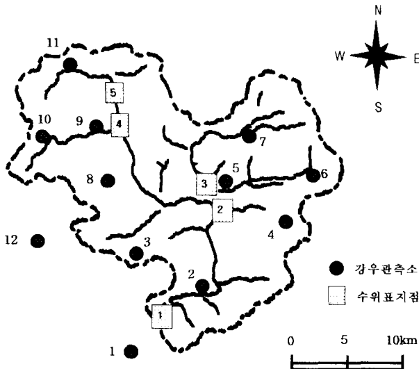
그림 3. 보청천 유역도
