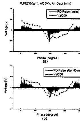
그림 9 AC 5kV에서 PD 패턴과 공극전압의 비교 (a) 초기 (b) 40분 후
