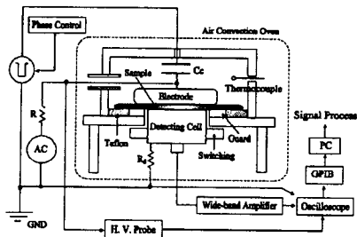
그림 2 교류전압 하에서의 측정시스템의 개략도 Fig. 2 Schematic diagram of measuring system
