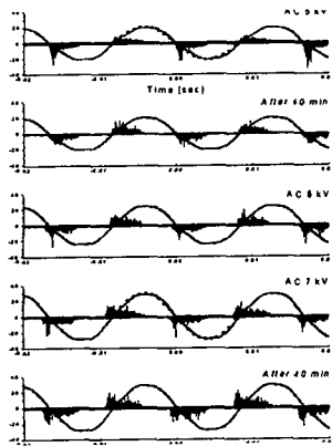
그림 4(b) 인가전압에 따른 PD 패턴의 변화 Fig. 4(b) Variation of PD patterns according to applied voltage
