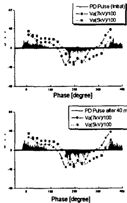
그림 11 AC 7kV에서 PD 패턴과 공극전압의 비교 (a) 초기 (b) 40분 후
