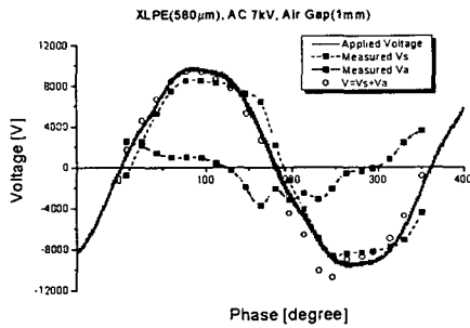
그림 10 AC 7kV에서 공간전하에 의한 전압분포(Vs:시료전압, Va:공극전압)
