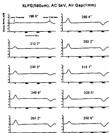
그림 5(a) AC 5kV에서 위상에 따른 공간전하분포 Fig. 5(a) Space charge distributions at AC 5kV according to phase
