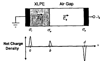
그림 6 공기층이 존재할 때 각 계면의 전하분포 Fig. 6 Charge density of each interface when air gap exists
