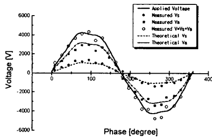
그림 7 AC 3kV에서 공간전하에 의한 전압분포( V_s :시료전압, V_a :공극전압)
