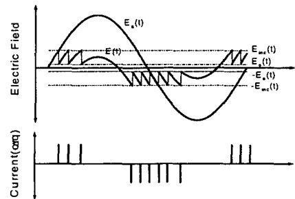
그림 1 전형적인 부분방전 패턴 Fig. 1 Typical pattern of partial discharge
