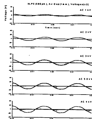
그림 4(a) 인가전압에 따른 PD 패턴의 변화 Fig. 4(a) Variation of PD patterns according to applied voltage
