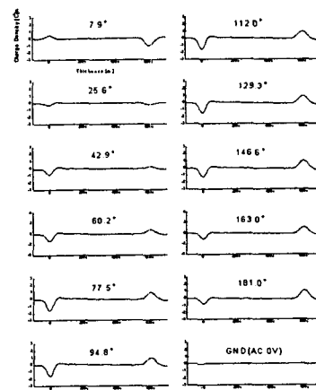
그림 5(b) AC 5kV에서 위상에 따른 공간전하분포 Fig. 5(b) Space charge distributions at AC 5kV according to phase
