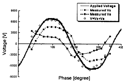
그림 8 AC 5kV에서 공간전하에 의한 전압분포( V_s :시료전압, V_a :공극전압)
