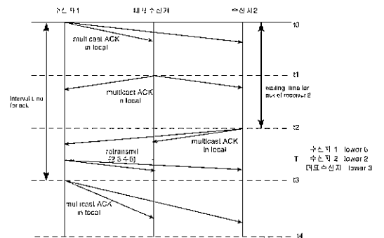
(그림 5) 지역 네트워크에서의 재전송
