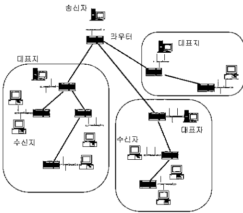
(그림 1) RMTP 구조
