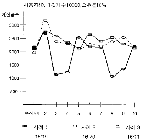
(그림 9) 패킷 수의 변화에 의한 재전송 횟수
