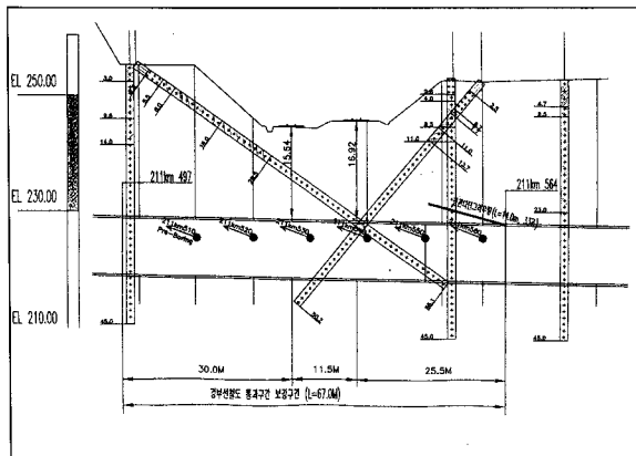
그림 8. 경부선 철도통과구간 보강
