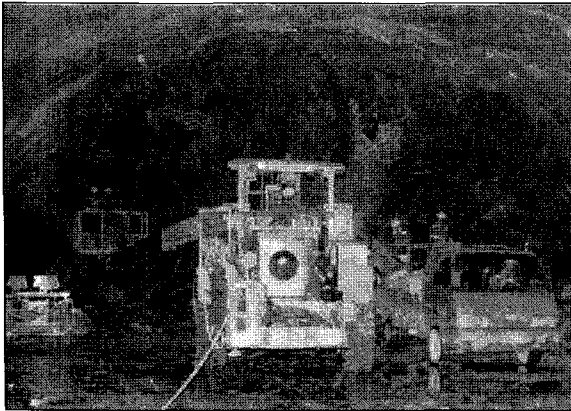
사진 8. 터널막장에서 장약
