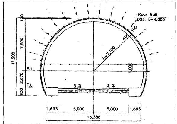
그림 2. 본선터널 표준지보패턴(P-2)
