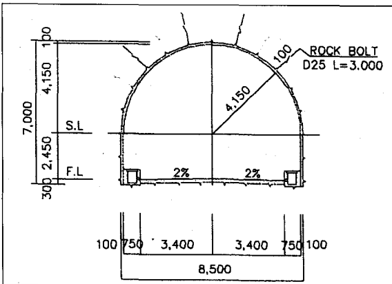
그림 3. 사갱터널 표준지보패턴(P-2)
