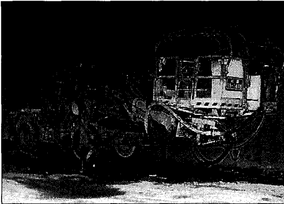
사진 11. 슛크리트 타설기
