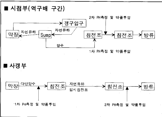
그림 9. 터널용수처리 계통도
