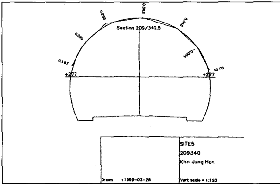
그림 5. 터널내공단면 측정결과
