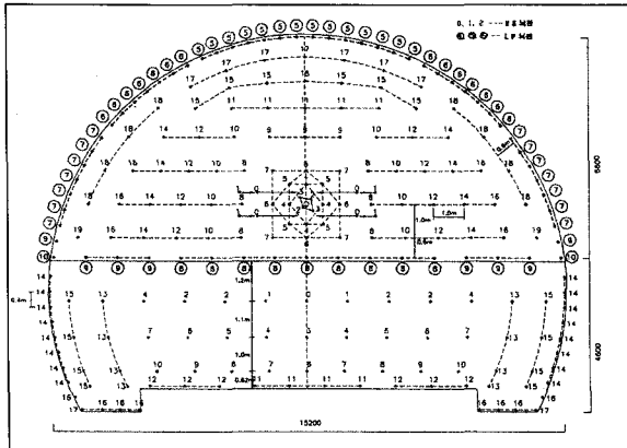
그림 7. 발파패턴도(P-2)
