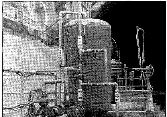
사진 14. 터널용수 중화처리장
