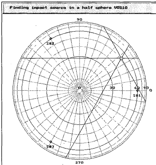
그림 10. 반구형에서의 충격점과 위치 추정치 비교 Fig.10. Comparison of the impact point and estimation point in spherical coordinate
