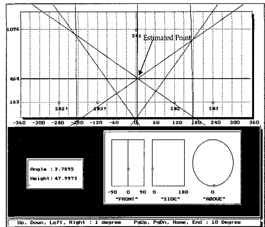
그림 9. 원통형에서의 충격점과 위치 추정치 비교
