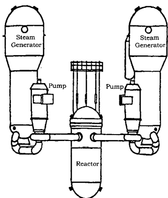
그림 1. NSSS의 가속도계 센서위치
