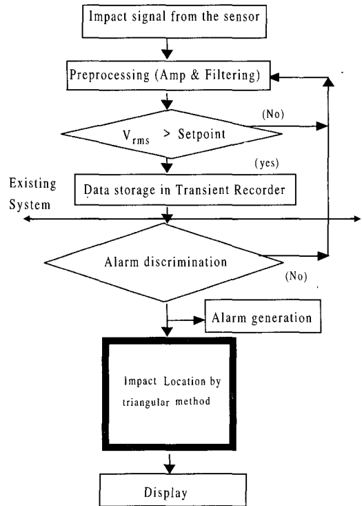
그림 4. 전체 알고리즘 흐름도
