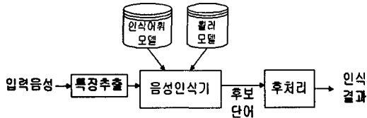
(그림 1) 인식대상 단어구별 시스템
