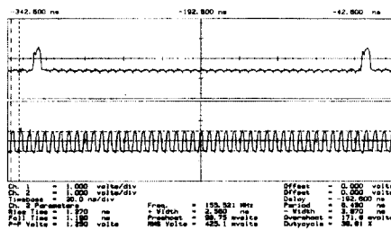
그림 3. 전압제어발진기의 출력 특성.
