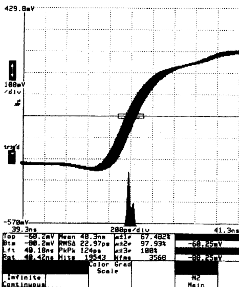
그림 4. 전압제어발진기의 지터 특성.
