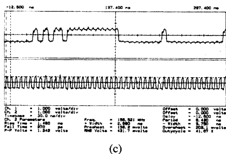
그림 2. ASIC 측정 결과 (a) 자유 동작, (b) 루프 2, (c) 루프 1.
