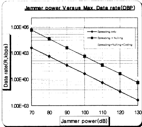
그림 7. OBP시스템 성능분석도
