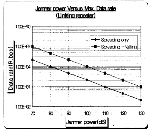
그림 4. Limiting repeater시스템 성능분석도
