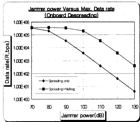
그림 5. Onboard Despreading성능분석도
