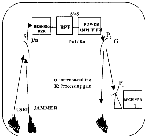
그림 2. Onboard Despreading중계시스템구성도
