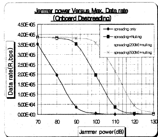
그림 6. Onboard Despreading성능분석비교도
