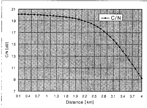
그림 7. 간섭에 의한 C/N의 열화(강우감쇄 고려시)
