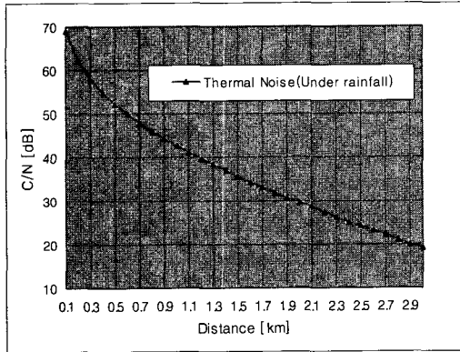
그림 6. 열잡음에 의한 C/N의 열화
