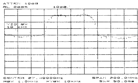
그림 10. C/I=15 dB에서 수신 스펙트럼
