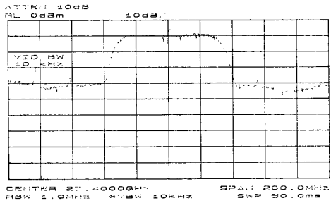
그림 9. C/I=17 dB에서 수신 스펙트럼
