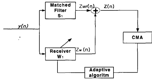
그림 3. 제안된 블라인드 다중사용자 검출기.
