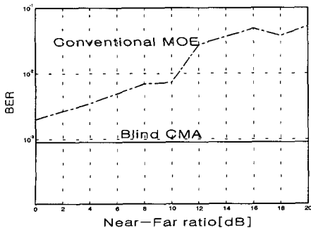
그림 8. NFR (0~20[dB]) 일 때 에러확률.
