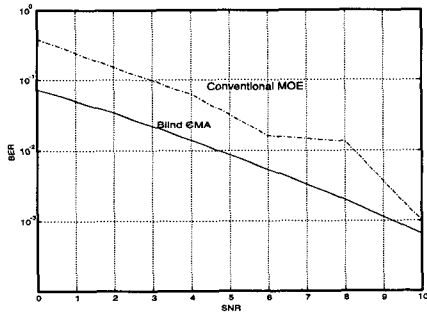
그림 7. SNR에 대한 BER ( k=8 ).
