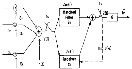
그림 2. 기존의 블라인드 MOE 다중 사용자검출기.
