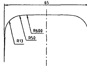
(a) 60kg 레일
