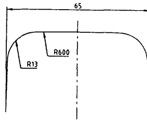
(b) R=600을 R=13까지 연장한 경우의 레일
