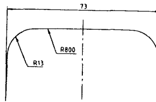
(c) R=800을 R=13까지 연장한 경우의 레일
