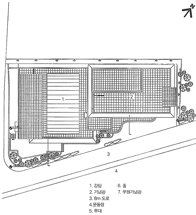
배치도
