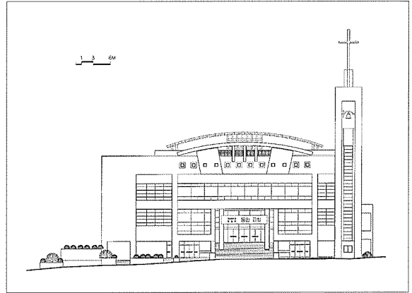
동안교회 정면도
