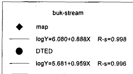
그림 11. 하천차수와 누적하천평균연장에 대한 분석(북천 유역)
