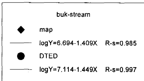
그림 8. 하천차수와 하천수에 대한 분석 (북천 유역)
