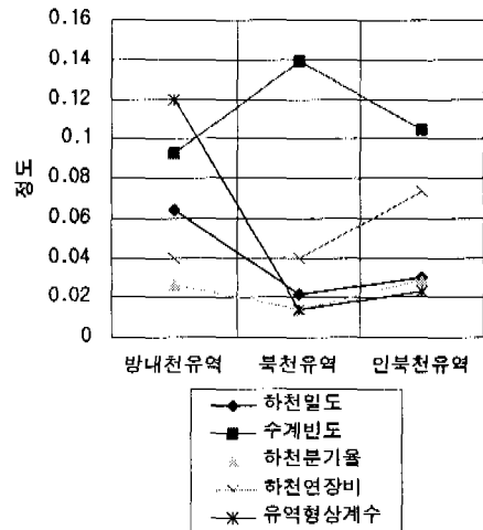
그림 13. 각 유역의 하천 형태학적 특성인자에 대한 정도 분포
