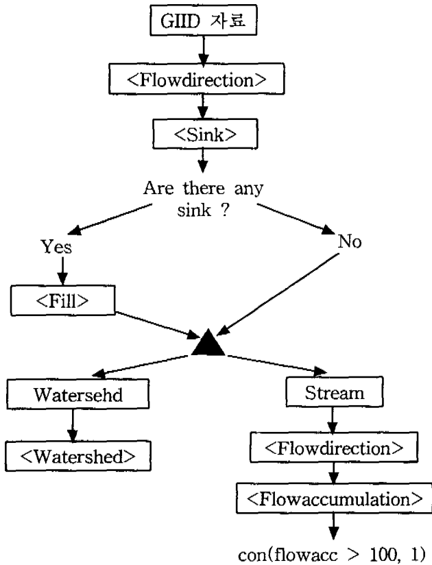
그림 3 수계망 및 유역 추출 과정
