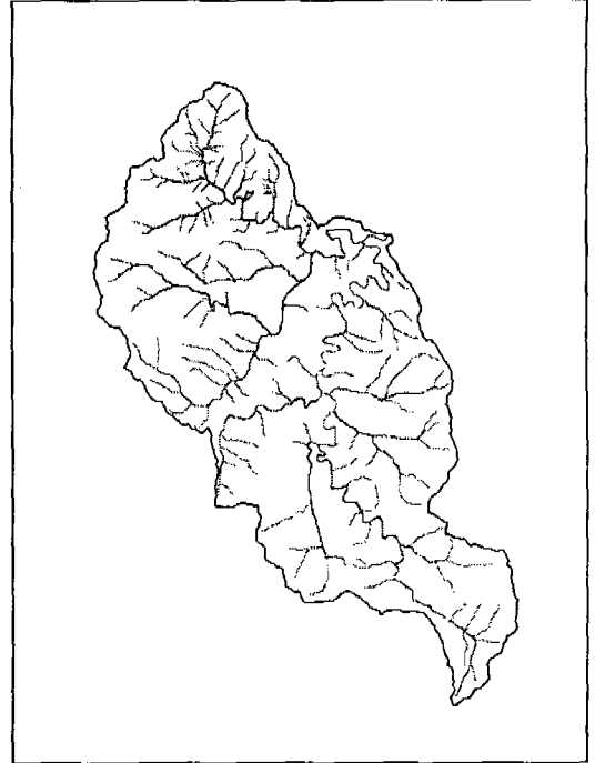
그림 4. 지형도를 수치화한 수계와 유역 (방내천)
