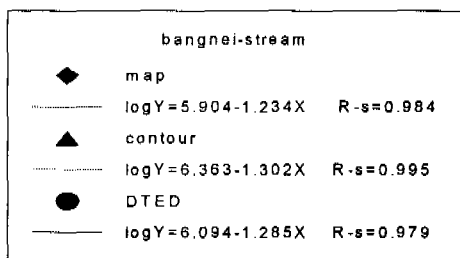
그림 7. 하천차수와 하천수에 대한 회귀분석 (방내천 유역)
