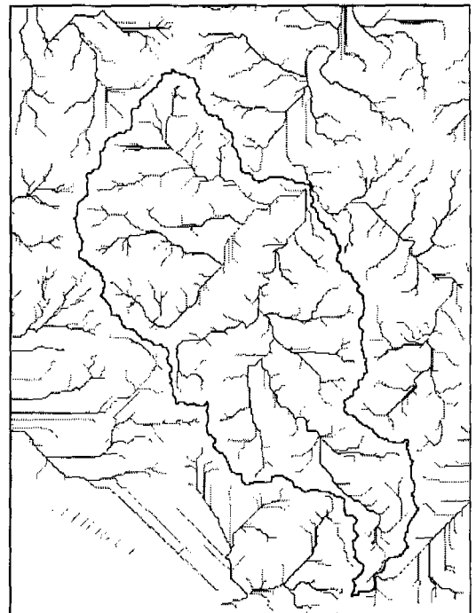
그림 5. 등고선을 변환한 그리드에서 추출한 수계와 유역 (방내천)
