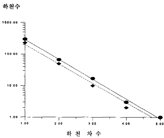
그림 7. 하천차수와 하천수에 대한 회귀분석 (방내천 유역)
