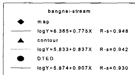
그림 10. 하천차수와 누적하천평균연장에 대한 분석 (방내천 유역)
