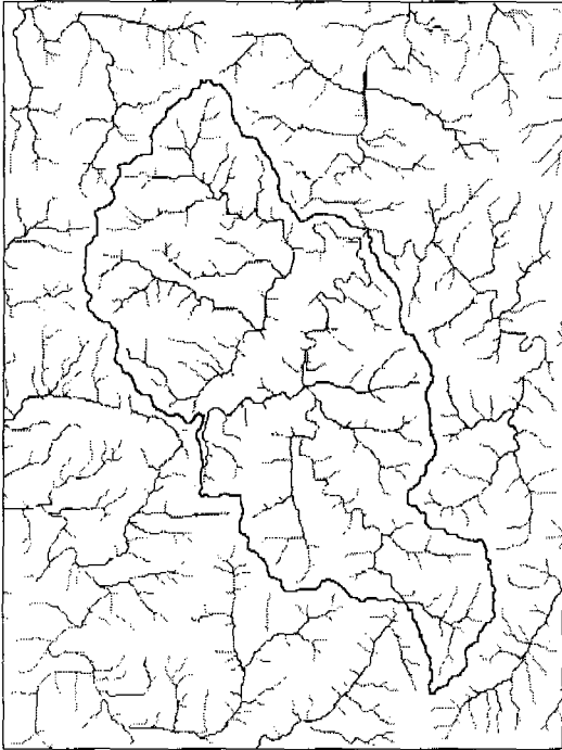
그림 6. DTED에서 추출한 수계와 유역 (방내천)
