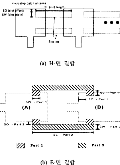
그림 4. 일차원 슬롯라인 결합구조 Fig. 4 One-dimensional slotline coupling structure (a) H-plane coupling (b) E-plane coupling
