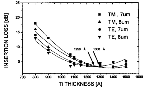
그림 15. 전체삽입손실. Fig. 15. Total insertion loss.
