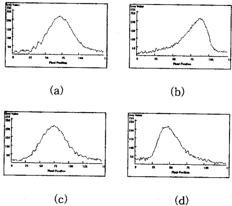
그림 13. 모드 형태. (a) TM, 횡모드 (b) TM, 종모드 (c) TE, 횡모드 (d) TE, 종모드 Fig. 13. Mode profiles. (a) TM, horizontal (b) TM, vertical (c) TE, horizontal (d) TE, vertical mode
