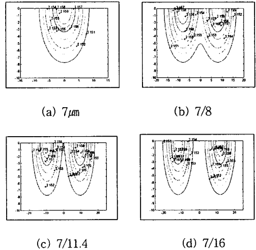
그림 16. z-cut Ti:LiNbO 3 굴절율 분포(폭/간격). (a) single channel region. (b) Mach-Zehnder Taper region (c) Mach-Zehnder Taper region (d) Mach-Zehnder parallel region
