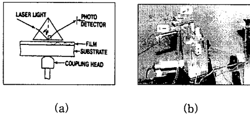
그림 9. 프리즘 커플러 구성.
