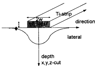
그림 4. Ti:LiNbO 3 광도파로.
