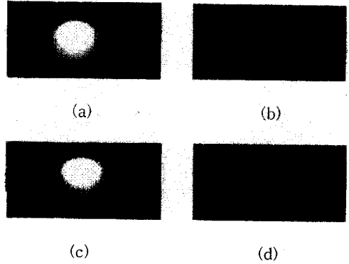
그림 12. 근거리 패턴. (a) TM/TM (b) TM/TE (c) TE/TE (d) TE/TM Fig. 12. Near field pattern. (a) TM/TM (b) TM/TE (c) TE/TE (d) TE/TM
