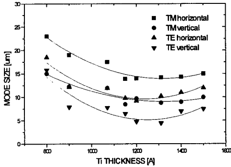
그림 14. 모드크기 Fig. 14. Mode size
