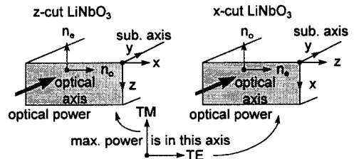
그림 6. 기관 및 광 축.
