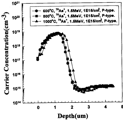
그림 2. 이온주입후 2단계 열처리조건( X°C, 10hrs + 1000°C, 5hrs, N 2 분위기)에 따른 반송자 농도를 SRP로 측정 한 결과. (a) 에피탁살 웨이퍼 (b) p-type 웨이퍼.
