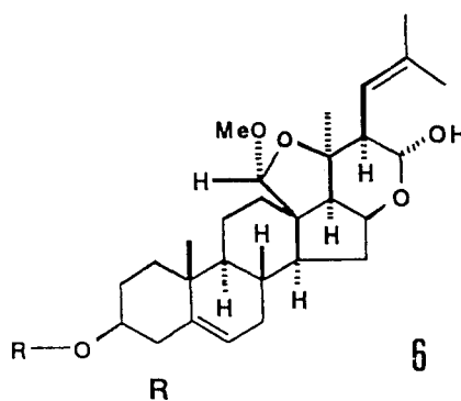
4-O- p -methoxybenzoyl-Rha-(1→2)-Glc
