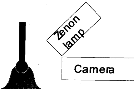
Fig. 5 제논 램프법을 이용한 금속 이행의 관찰법. 하는데 비하여, 액적 형상을 직접 관찰하기 때문에
