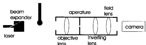
Fig. 4 Laser Back Lightening법의 모식도.
