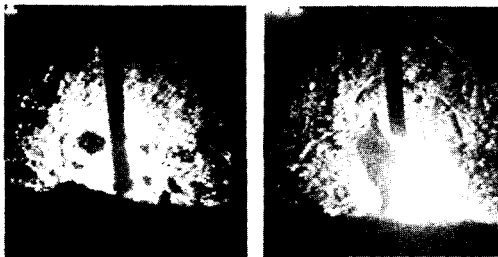
Photo. 9 천이 이행 모드에서의 스패터 발생. (a) 단락 이행시의 스패터 발생, (b) 입상 이행에서의 스패터 발생
