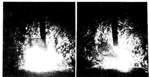
Photo. 6 CO 2 용접에서 실제 입상 이행 과정
