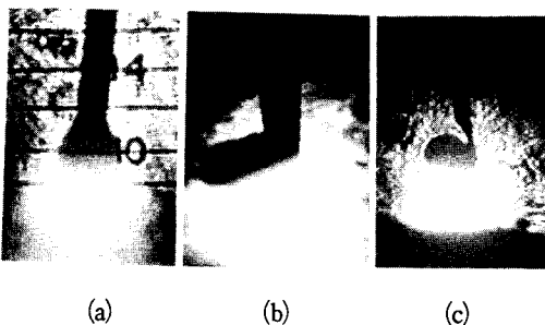
Photo. 1 보호가스의 종류에 따른 용접 아크의 특성 (a) 아르곤, (b) 헬륨, (c) CO 2
