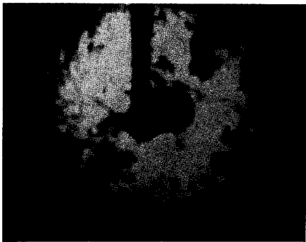
Photo. 5 CO 2 용접에서 액적이 repelling되는 현상
