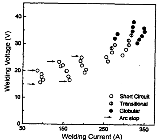
Fig. 6 CO 2 용접에서 용접 전류에 따른 금속 이행 모드의 변화.
