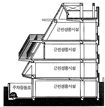
횡단면도
