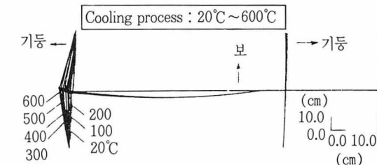
(그림 6) 가구(架構)의 열변형(냉각시)
