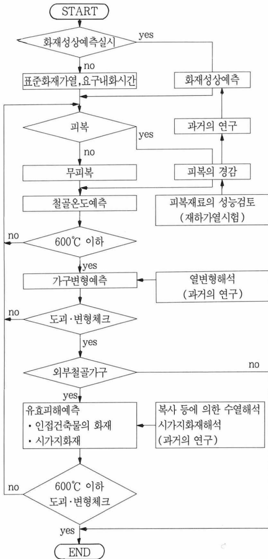
(그림 4) 내화강을 이용한 건물의 내화설계 Flow
