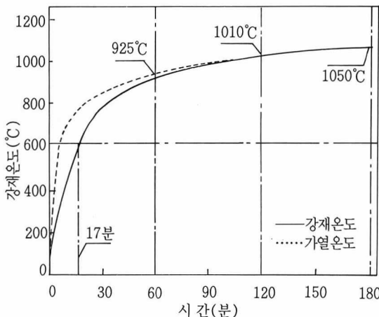
〈그림 1〉 표준가열곡선과 무피복 철골의 온도상승
