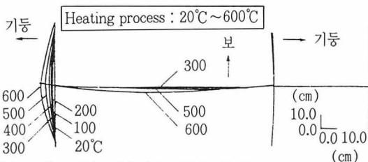
(그림 5) 가구(架構)의 열변형(승온시)
