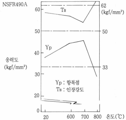
〈그림 8〉 내화강의 가열 후 강도
