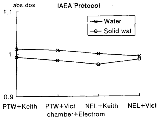
그림 6. PTW+Keithley, water에 정규화한 6MV 광자선의 상대 흡수선량 비교
