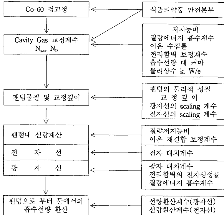
그림 1. 흡수선량 교정 과정
