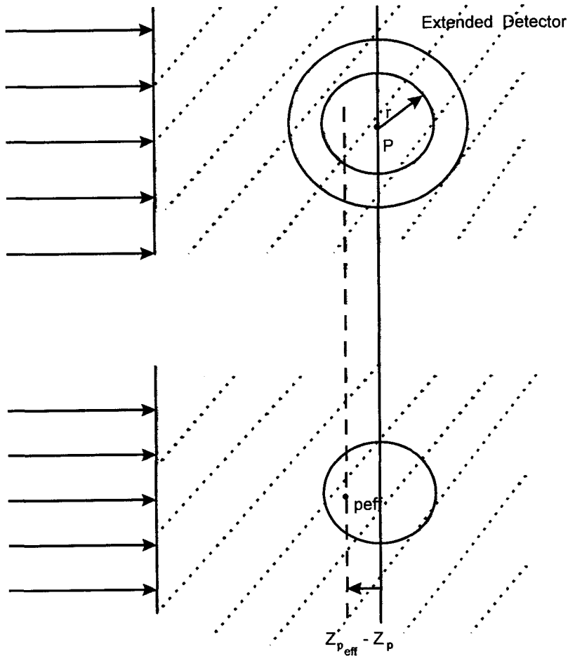
그림 4. 전리함 중심으로부터 유효측정점의 이동( Z_{p_{eff}} - Z_p = 0.75r )
