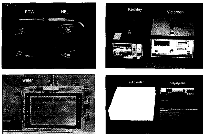
그림 2. 측정기구 및 측정팬텀
