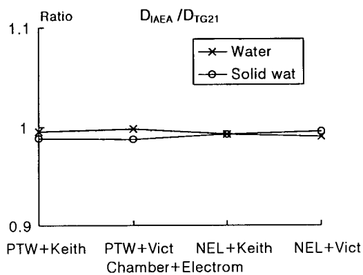
그림 5. 물팬텀, 고체물팬텀에서 6MV 광자선의 흡수선량 비교
