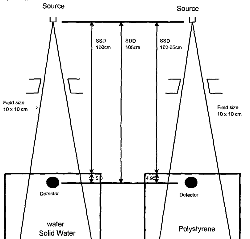
그림 3. 선량측정을 위한 기하학적 조건
