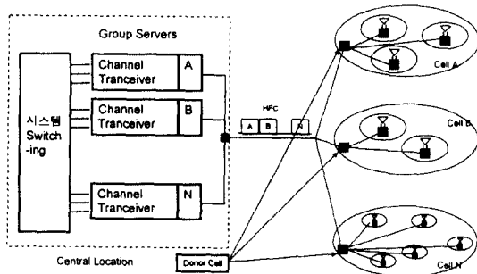
그림 1. 분산 안테나 시스템 Fig. 1 Distributed Antenna Systems
