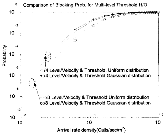
그림 18. 멀티레벨 임계값 핸드오프알고리즘의 블러킹 확률비교 Fig. 18. Comparison of blocking prob. of multi-level threshold handoff algorithm
