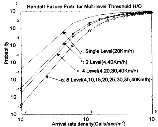
그림 12. 멀티레벨 임계값 핸드오프알고리즘의 핸드오프 실패 확률(1)
