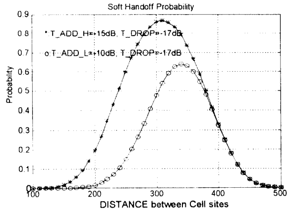
그림 2 소프트 핸드오프 발생 확률 Fig. 2. Soft handoff probability
