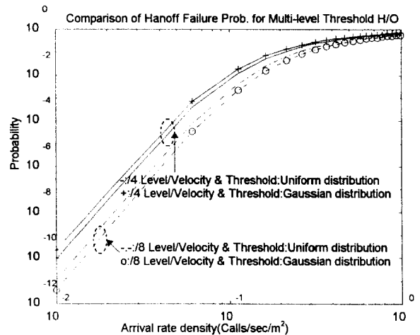
그림 19. 멀티레벨 임계값 핸드오프알고리즘의 핸드오프 실패확률비교 Fig. 19. Comparison of handoff failure prob. of multi-level threshold handoff algorithm
