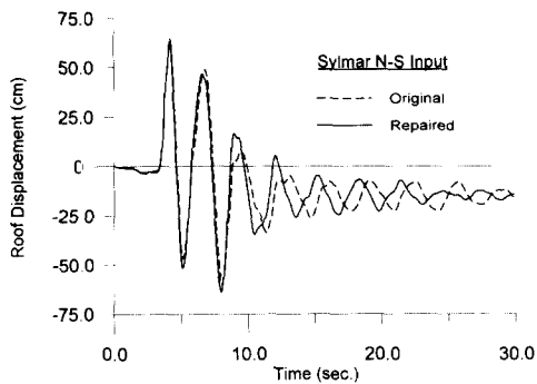
그림 14 지붕변위 시각력
