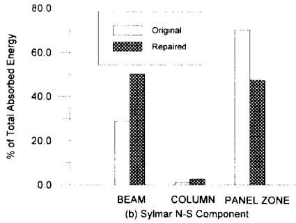
그림 19 구조물 내의 에너지소산 패턴 비교
