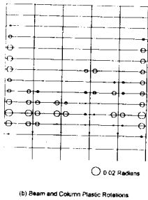
그림 17 패널 존, 보, 및 기둥의 최대소성 회전각 (보강구조물의 Sylmar N-S 가속도 성분에 대한 응답)
