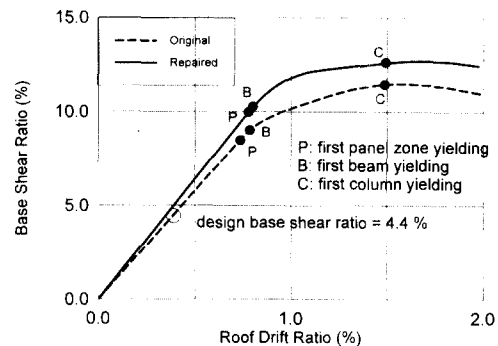
그림 9 푸쉬오버 해석 결과 비교
