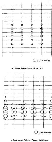
그림 11 패널존, 보, 및 기둥의 최대 소성 회전각 (원구조물의 지붕형변위비가 2%에 이르도록 푸쉬 오버 했을 때)
