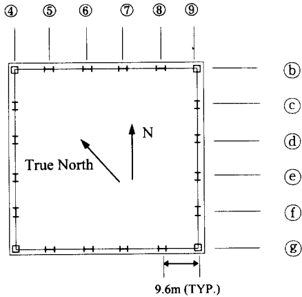
그림 3 구조평면 개요
