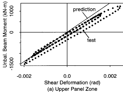
그림 7 불균형 보 휨모멘트와 이중패널존의 환선회전각 관계 (Lee-Uang 1997)
