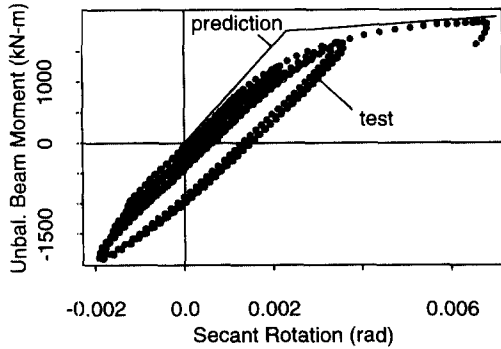
(c) Dual Panel Zone 그림 8 예측값과 시험결과와의 비교 (Lee-Uang 1997)
