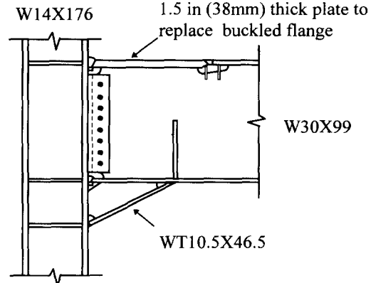
그림 1 현치로 보강된 철골 모멘트 접합부 (Uang-Bondad 1996a)
