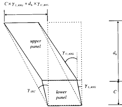
그림 6 이중패널존의 전단변형 양상 (Lee-Uang 1997)
