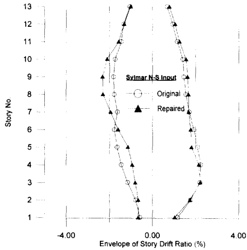
그림 15 층간변위 비교
