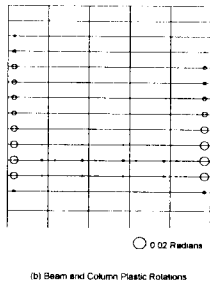
그림 16 패널 존, 보, 및 기둥의 최대소성 회전각 (원구조물의 Sylmar N-S, 가속도 성분에 대한 응답)
