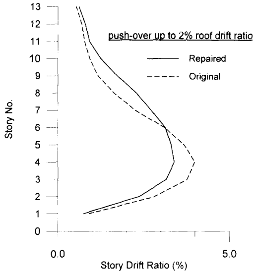
그림 10 층간변위 비교
