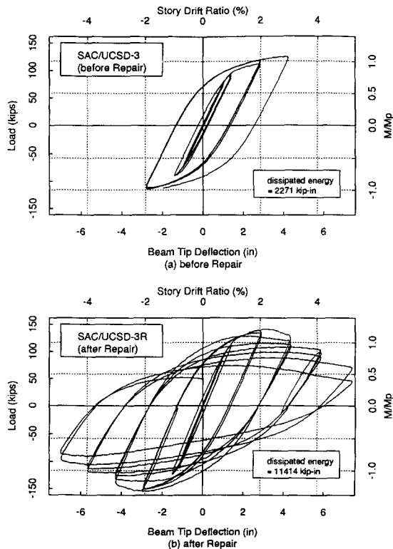
그림 2 보강 전후의 보-기둥 부분골조의 이력거동 비교 (Uang-Bondad 1996a)
