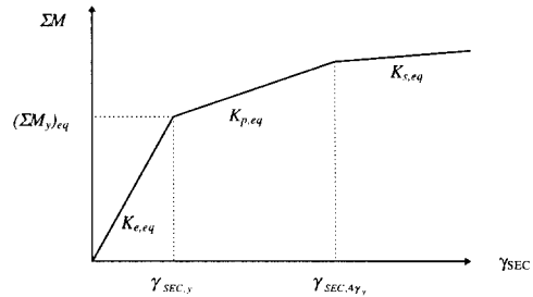
그림 7 불균형 보 휨모멘트와 이중패널존의 환선회전각 관계 (Lee-Uang 1997)
