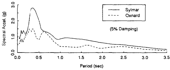
그림 13 입력 지진동 (1994년 Northridge 지진)
