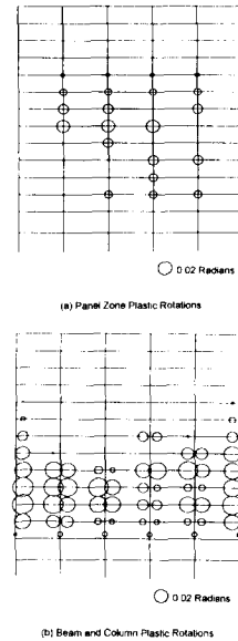
그림 12 패널존, 보, 및 기둥의 최대 소성 회전각 (보강구조물의 지붕형변위비가 2%에 이르도록 푸쉬 오버 했을 때)
