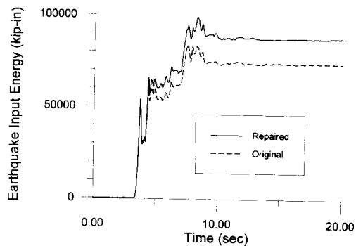
그림 18 입력 지진에너지의 시각력 비교
