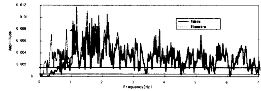
(d) Comparison of Fourier transform
