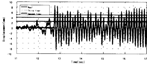
그림 9 Overlaid global response time history(PGA 0.319g)
