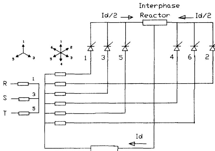
Fig. 2 Thyristor rectifier circuit.
