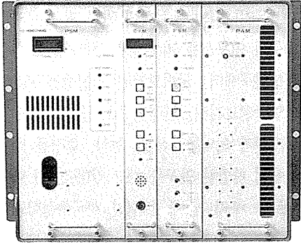
▲ 무선호출 송신기(대출력)
