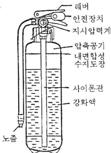
[그림 1] 강화액소화기 구조 단면도
