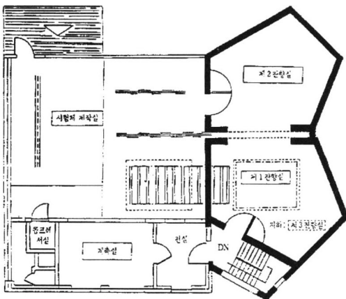
[그림 1] 방재시험연구소 음향시험동 개요도
