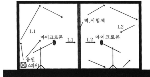
[그림 2] 음향투과손실측정 개요도
