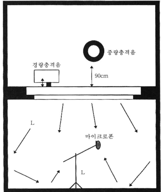
L: 바닥충격음레벨(dB)
