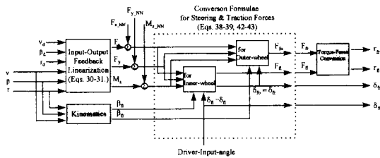
그림 5. 우측 회전을 기준으로한 조향과 추진력 제어의 블록도 Fig. 5. Block Diagram of Control for Steering and Traction In Right-Turn.
