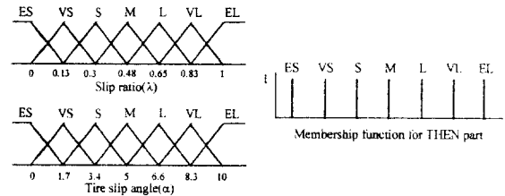
그림 7. 횡축력 추정을 위한 소속 함수 Fig. 7. Membership Functions for the Cornering Force Estimation.
