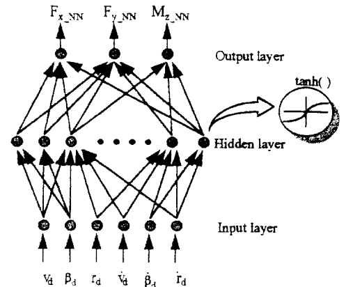
그림 6. 3 - 계층 신경 회로망 보상기의 구조 Fig. 6. Structure of 3-layer Neural Network Compensator.
