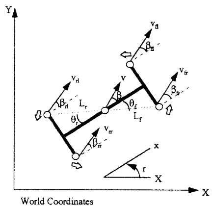
그림 2. 국부 속도 벡터 들의 기구학적 관계
