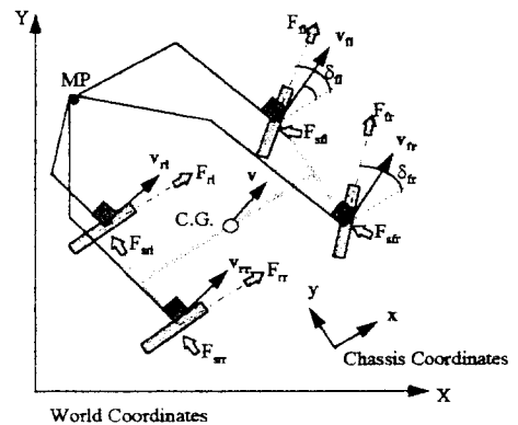
그림 1. 전기 자동차 모델. among local velocity vector
