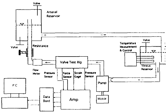
그림 1. 실험 장치 구성도 Fig. 1. Schematic diagram of the experimental apparatus
