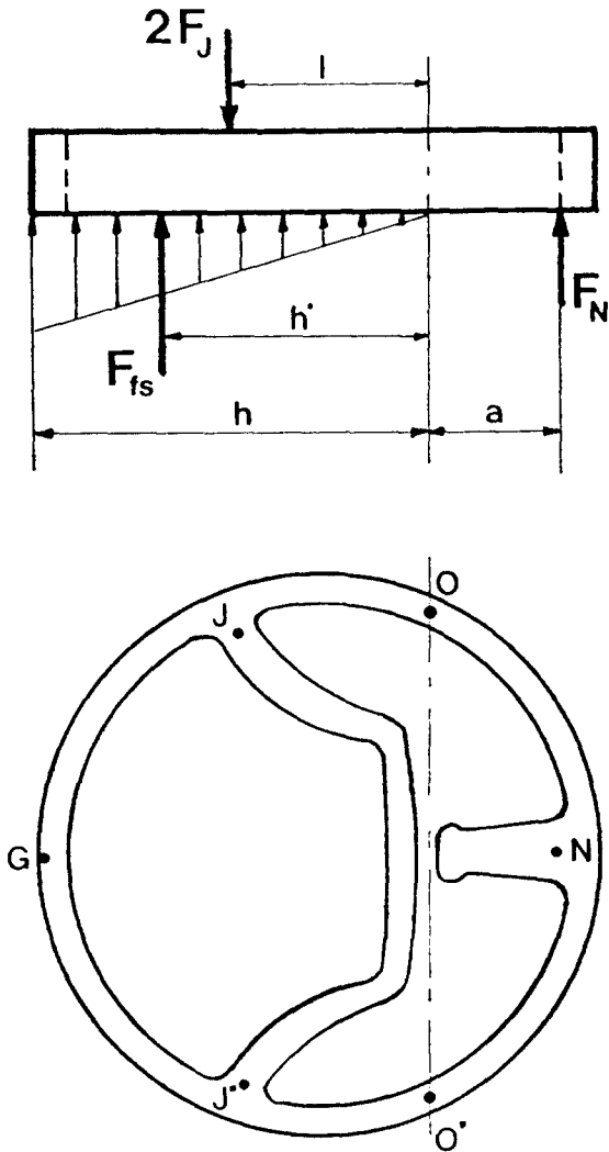
그림 5. 충격시 링과 포스 센서간의 반력 관계도 Fig. 5. Schematic diagram showing reaction forces between the ring and the force sensor during impact
