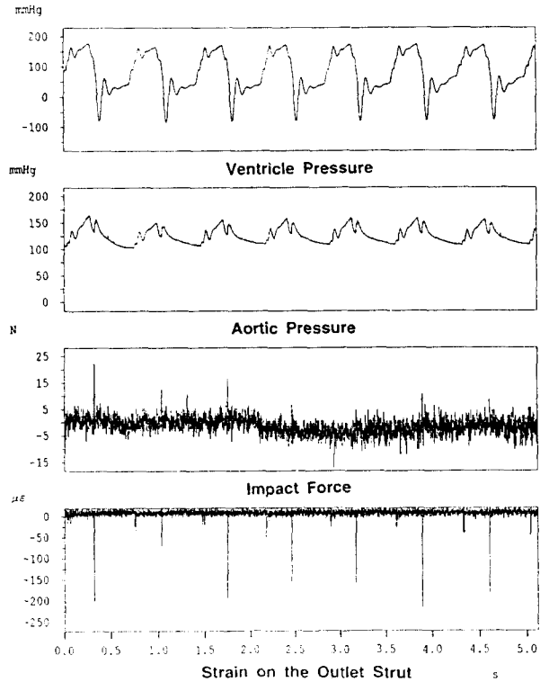
그림 6. 압력, 충격력, 변형률 실험결과 Fig. 6. Experimental results showing pressures, impact force and strain
