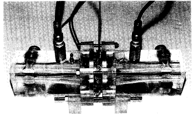
그림 2. 밸브 설치 고정구의 사진과 구성도 Fig. 2. Photograph and schematic diagram of a valve setting rig
