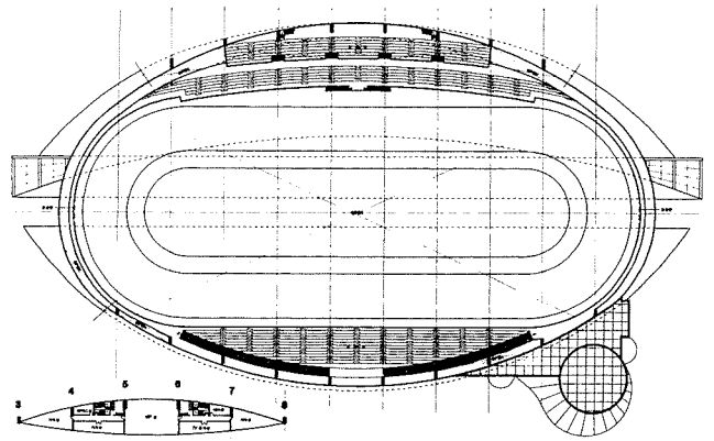
3층 평면도
