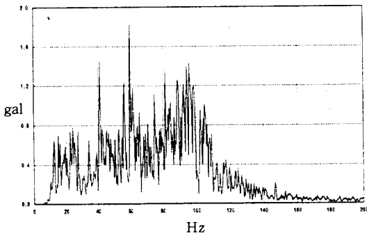
그림 19. 기차하중에 대한 가속도스펙트럼
