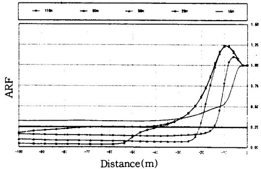
그림 11. 보강폭에 따른 진폭감소계수의 변화 : 20Hz
