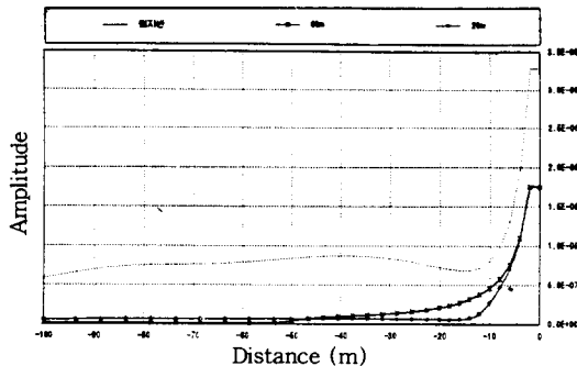
그림 14. 보강폭에 따른 진폭변화 : 20Hz
