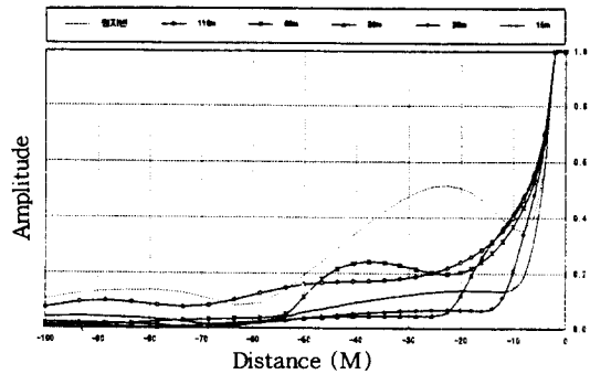
그림 12. 보강폭에 따른 진폭변화 : 50Hz
