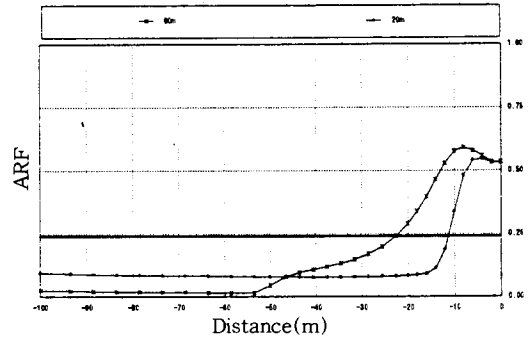
그림 15. 보강폭에 따른 진폭감소계수의 변화 : 20Hz
