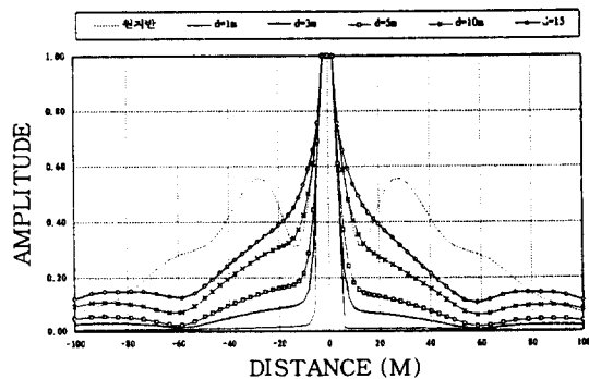
그림 5. 보강깊이에 따른 진폭변화 : 50Hz
