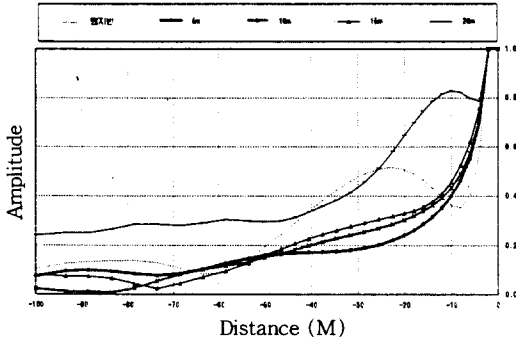
그림 9. 보강길이에 따른 진폭변화 : 50Hz
