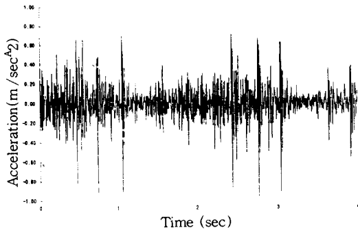
그림 18. 기차하중에 대한 시간이력곡선
