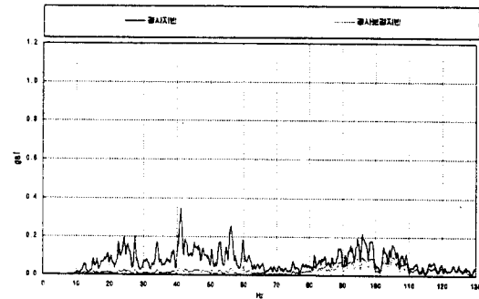
그림 21. 기차하중이 작용할때 50m지점의 가속도스펙트럼
