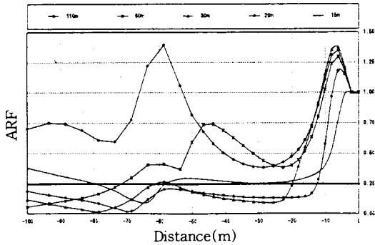
그림 13. 보강폭에 따른 진폭감소계수의 변화 : 50Hz
