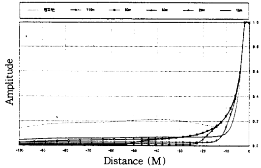
그림 10. 보강폭에 따른 진폭변화 : 20Hz
