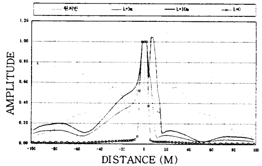
그림 7. 기초중앙에서 수신부까지의 거리에 따른 진폭변화 : 50Hz
