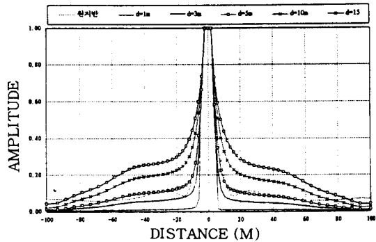
그림 4. 보강깊이에 따른 진폭변화 : 30Hz
