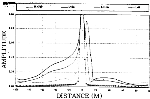
그림 6. 기초중앙에서 수신부까지의 거리에 따른 진폭변화 : 30Hz
