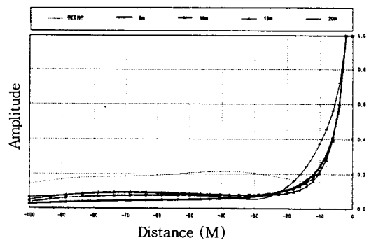
그림 8. 보강깊이에 따른 진폭변화 : 20Hz
