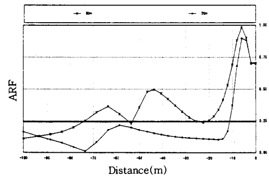
그림 17. 보강폭에 따른 진폭감소계수의 변화 : 50Hz
