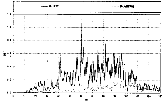
그림 20. 기차하중이 작용할때 25m지점의 가속도스펙트럼
