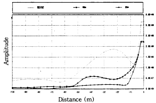
그림 16. 보강폭에 따른 진폭변화 : 50Hz
