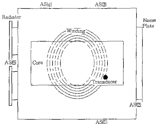
그림 8. 초음파 탐촉자 및 권선과 철심사이의 초음파 발생장치 설치위치
