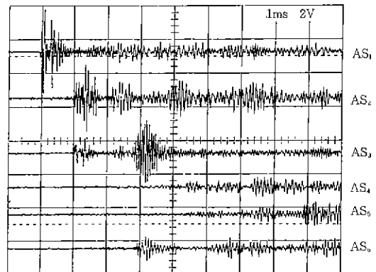
그림 7. 권선의 표면에서 발생한 초음파의 측정 파형 Fig. 7 The detection waves of the ultrasonic generated on the surface of the winding
