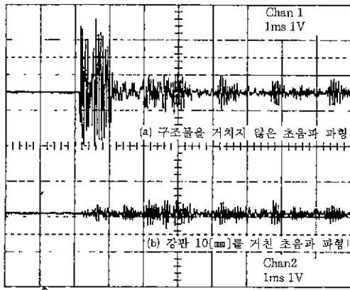
그림 4. 변압기 구조물에 의해 변형된 초음파 신호 Fig. 4. The ultrasonic signals interfered by materials of transformer
