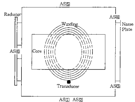
그림 6. 초음파 탐촉자 및 권선표면의 초음파 발생장치 설치위치 Fig. 6. Position of the ultrasonic detectors on the wall and the transducer on the winding
