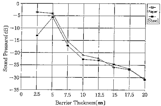
그림 5. 변압기 구조물에 의한 음압의 감쇄 Fig. 5. Attenuation of the sound pressure by materials of transformer
