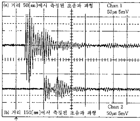
그림 3 초음파 발생장치와 탐촉자의 대향거리 변화에 따른 초음파 파형의 변화 Fig. 3. Ultrasonic wave variation with distance between the ultrasonic generator and detector
