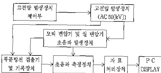
그림 1. 초음파 신호 측정 시스템의 개략도 Fig. 1 Schematic diagram of the ultrasonic signal detector
