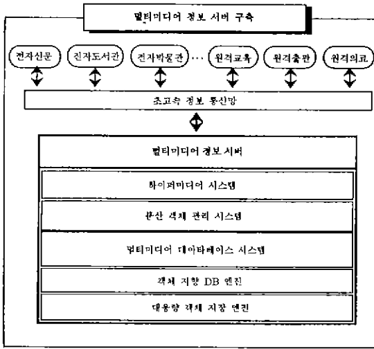
그림 1 멀티미디어 정보서버 아키텍처
