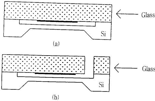
그림 2. (a) 절대압과 (b) 상대압 용량형 압력센서의 단면도
