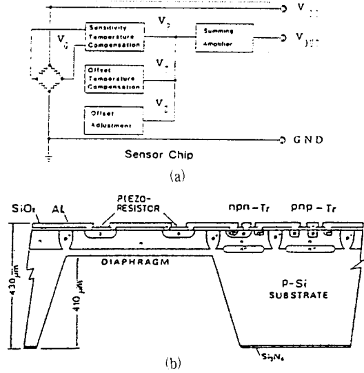
그림 6. 완전 집적화한 바이폴라 압력센서의 (a) 블록 다이어그램 및 (b) 단면도
