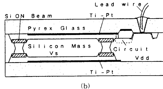
그림 13. 용량형 압력센서를 이용한 가속도 센서의 (a) 원리도 및 (b) 단면도
