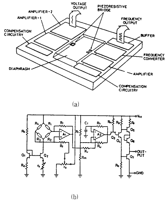
그림 3. 전압과 주파수 출력이 가능한 바이플라 집적화 압력센서의 (a) 도식적 다이어그램 및 (b) 주파수 출력용 신호처리 회로도
