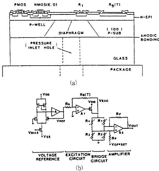
그림 5. CMOS 집적화 압력센서의 (a) 단면도 및 (b) 신호처리 회로도
