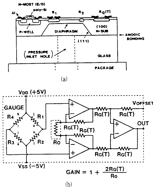
그림 4. NMOS 집적화 압력센서의 (a) 단면도 및 (b) 신호처리의 회로도
