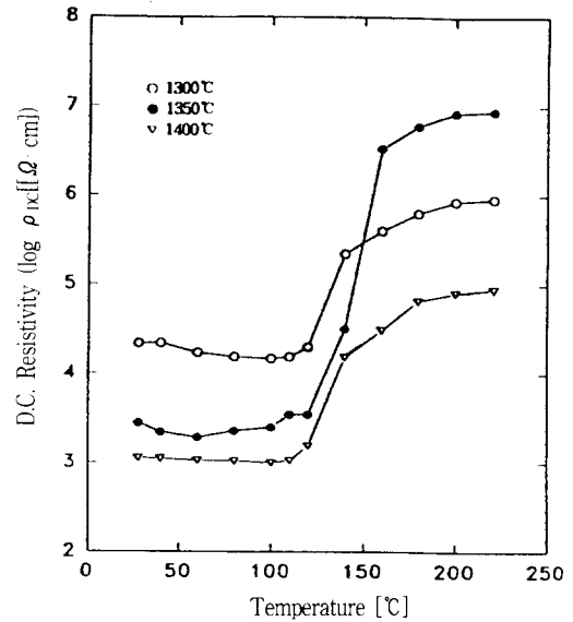
그림 5. 소결온도에 따른 온도 대 직류저항률 특성 ( TiO_2 과잉 : 0.02mol) Fig. 5. D.C. resistivity vs. Temperature characteristics at various sintering temperature( TiO_2 excess : 0.02mol).
