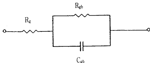
그림 7. 등가회로 모델
