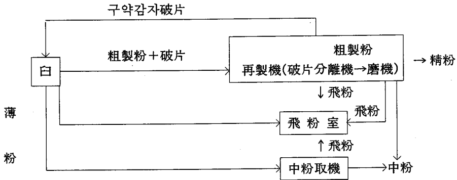
그림 5. 곤약 정분 가공공정도
