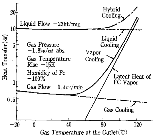
<그림3·2> 냉각방식에 따른 열전달 특성
