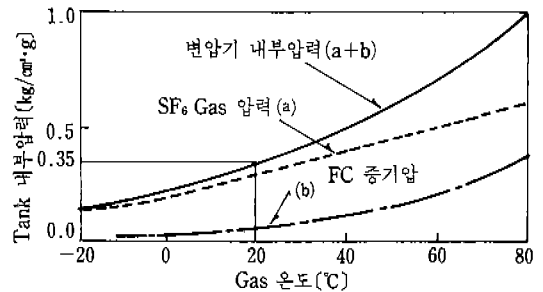
<그림4·2> SF 6 +FC의 압력상승의 온도 의존성
