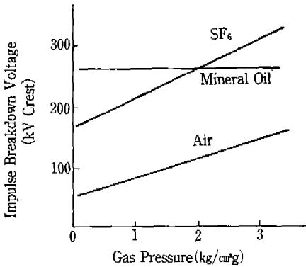
<그림5.2> SF 6 Gas의 충격전압 특성
