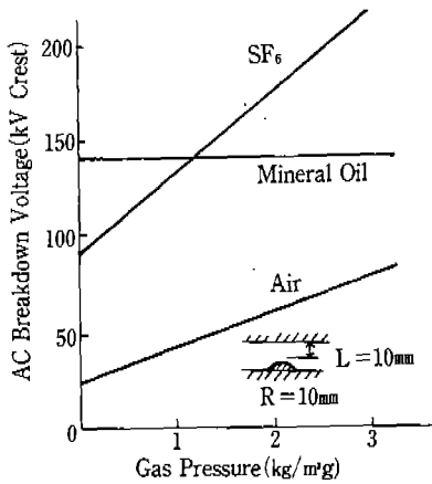
<그림5.1> SF 6 Gas의 AC 내전압 특성
