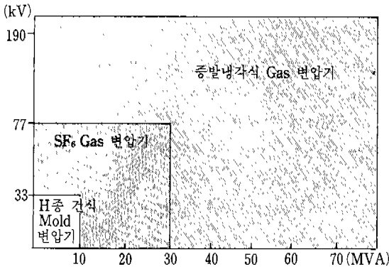
<그림 2·1> 불연성 변압기의 적용구분
