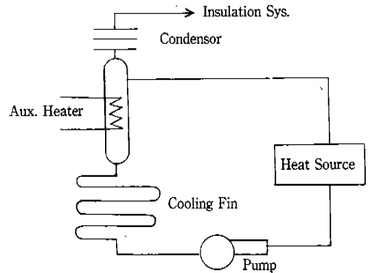
<그림4·1> 냉매의 Gas 방출 System
