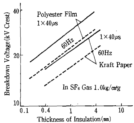
<그림5.3> PET, Kraft의 내전압 특성
