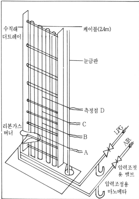
그림2 연료장치의 배관배열
