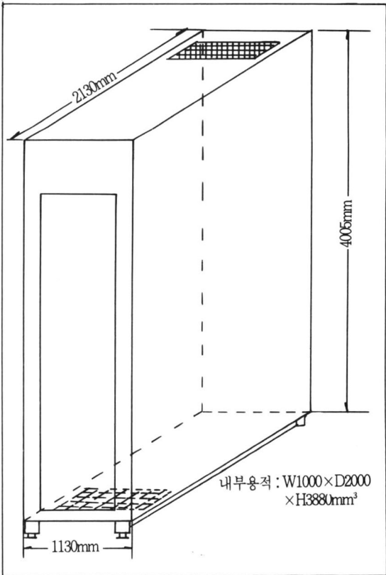
그림 1. 케이블 수직연소성 시험기
