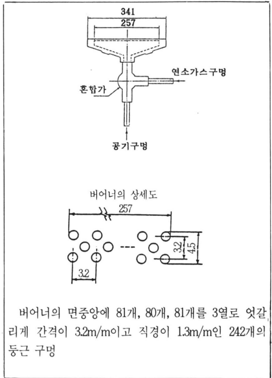
그림3 버너
