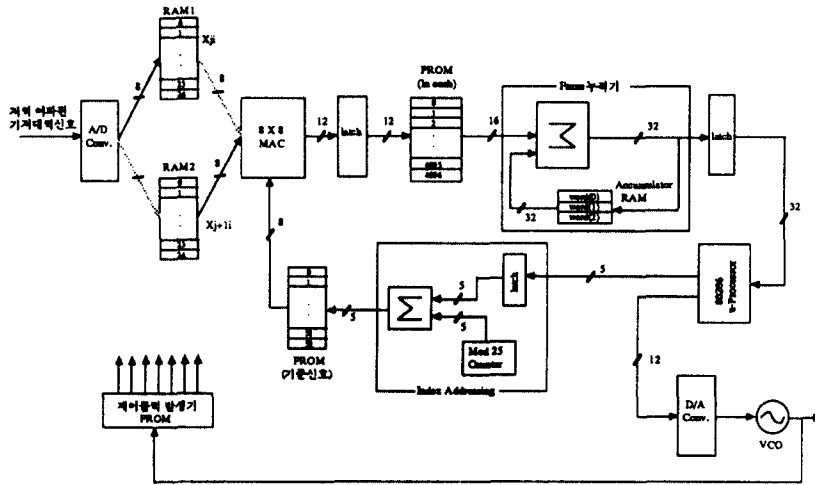
그림 3. 최적 동기 방식의 도플러 추적 장치 구성도 Fig. 3. Block diagram of the Doppler tracking system using the optimum synchronization techniques.
