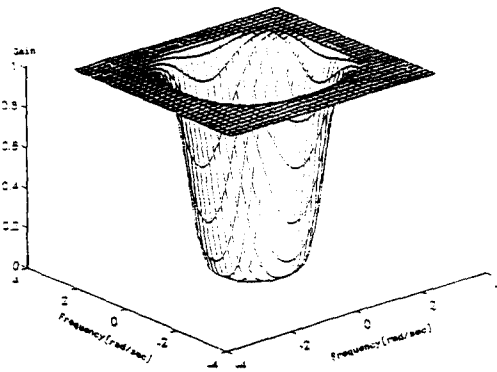
그림 13. 2차원 대역통과필터 Fig 13. Two-dimensional bandpass filter
