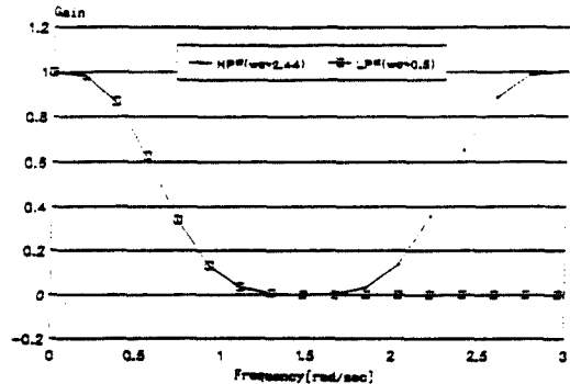
그림 8. 대역저지필터의 주파수응답 Fig 8. The frequency response of the band-reject filter
