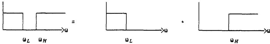
그림 6. 대역저지필터의 실현방법 Fig 6. The realized method for the band-reject filter
