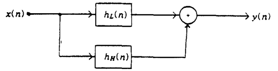
그림 7. 대역저지필터 실현을 위한 블록도 Fig 7. The block diagram for the band-reject filter
