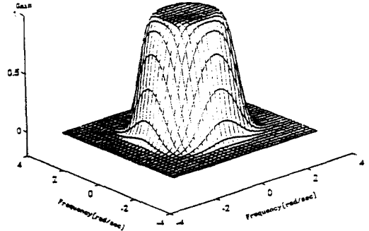
그림 11. 2차원 저역통과필터 Fig 11. Two-dimensional lowpass filter
