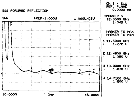
그림 9. 제작된 안테나의 Smith 도표와 VSWR(Type #3) Fig. 9. Smith chart and VSWR of the antenna(Type #3)
