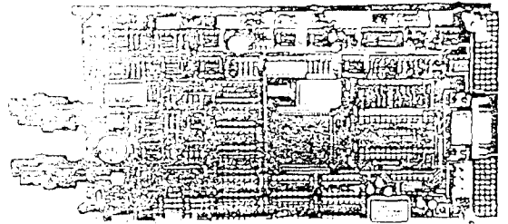
그림 12. 구현한 무선 모뎀 Fig. 12. Configuration of implemented MODEM
