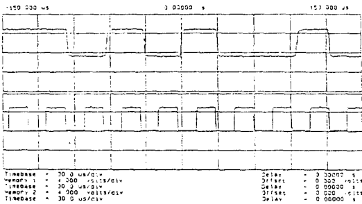
그림 22. 기저대역신호와 복원 클럭 Fig. 22. Baseband signal and recovered clock
