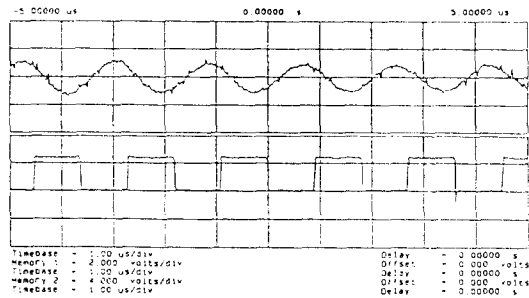
그림 18. 수신신호와 복원된 반송파 신호파형 Fig. 18. Received signal and recovered carrier signal
