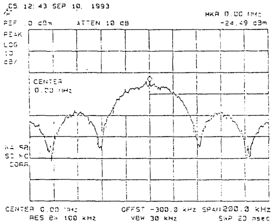
그림 13. 송신될 데이터의 스펙트럼 Fig. 13. Spectrum of data before transmission
