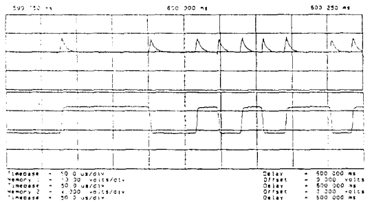
그림 20. edge 검출기의 출력신호와 복원된 데이터신호 Fig. 20. Output signal of edge detector and recovered data signal
