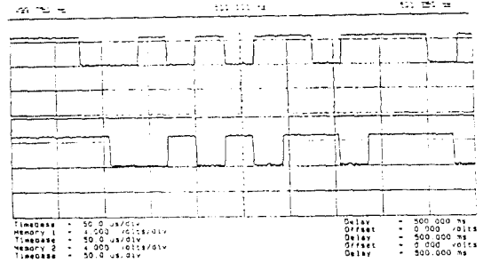
그림 24. 최종 송신 데이터신호와 최종 수신 데이터신호 Fig. 24. Transmitted data signal and receive data signal
