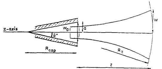
그림 1. 원뿔형 컬러케이트 혼 Fig. 1. Conical corrugated horn
