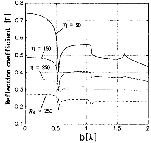
그림 5. 입사각 60도에서의 반사계수의 크기 ( a/b=0.25, \eta=50, 150, 250 및 R_0=250 [ \Omega/\text{square} ]) Fig 5. The magnitude of reflection coefficient for incident angle 60^\circ ( a/b=0.25, \eta=50, 150, 250 and R_0=250 [ \Omega/\text{square} ])
