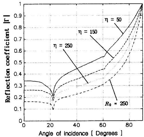
그림 6. 입사각에 따른 반사계수 ( h=0.3[\lambda], a=2h, b=1.6[\lambda] ) Fig 6. The reflection coefficient of the angles of incidence ( h=0.3[\lambda], a=2h, b=1.6[\lambda] )
