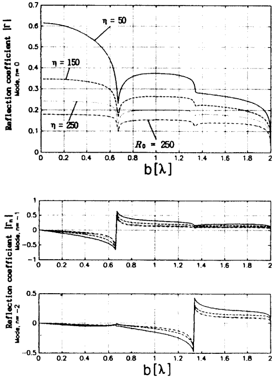
그림 4. 모드 n=0, -1 및 -2 에서의 반사계수 ( \phi=30^\circ, a/b=0.25, \eta=50, 150, 250 및 R_0=250 [ \Omega/\text{square} ]) Fig 4. The reflection coefficient for mode n=0, -1, \text{ and } -2 ( \phi=30^\circ, a/b=0.25, \eta=50, 150, 250 and R_0=250 [ \Omega/\text{square} ]) (Positive : Propagation Mode, Negative : Evanescent Mode.)
