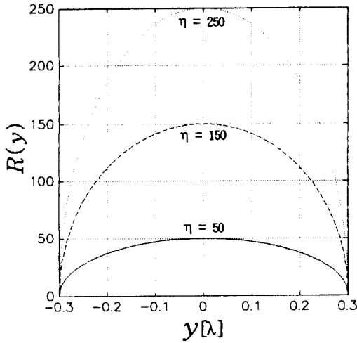
그림 2. 저항띠의 변하는 저항율 ( h = 0.3, -h \leq y \leq h )
