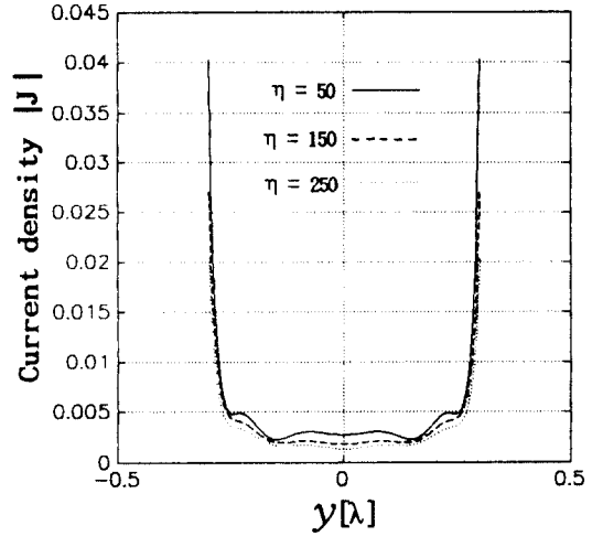
그림 3. 수직입사시 전류밀도의 크기, |J| ( h = 0.3[\lambda], a = 2h, b = 1.8a )
