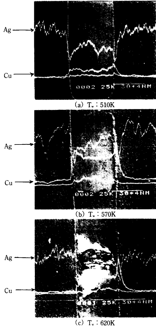
그림 11 Fracture surface of the bonds by Pulse Heat Tip process(Thick film side)
